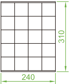
吸塑Blister-A(B)-310*240*20
