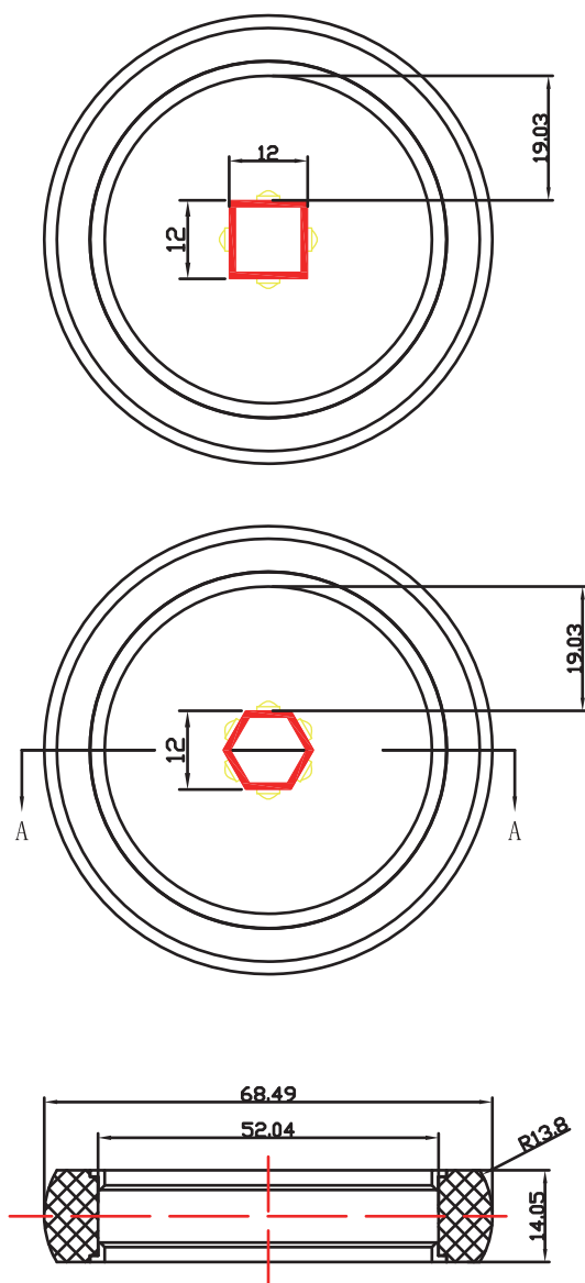
SECTION A-A
