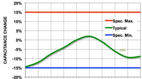
BME MINI SWITCHMODE TEMPERATURE COEFFICIENT
