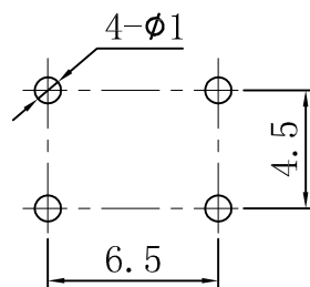
印制线路板开孔 P. C. B. HOLE DETAIL
