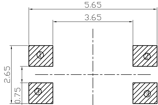
安装参考图
