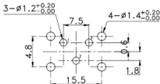
安装孔位图 Mounting Hole
