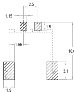
SMT type
